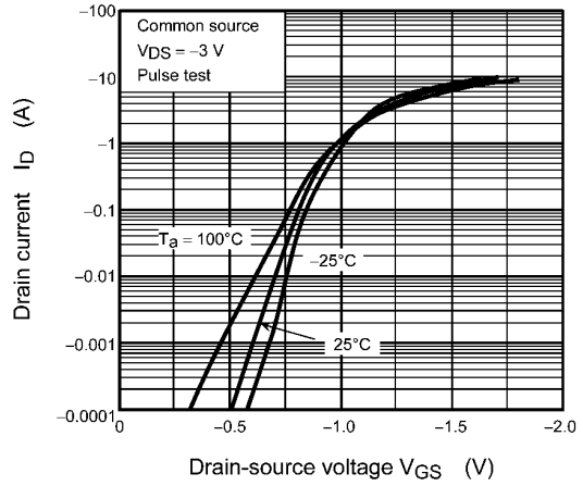
Fig. 7.2 I_D - V_{GS}
