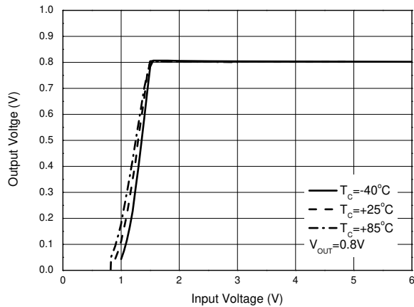
Output Voltage vs. Input Voltage (I OUT =300mA)
