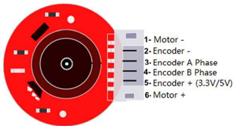
Pinmap
