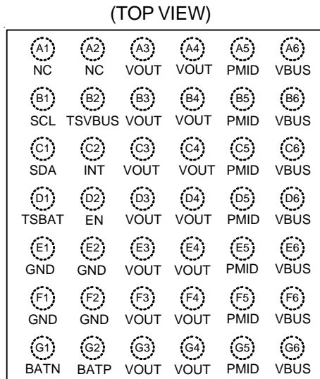
WL-CSP-42B 2.75x3.05 (BSC)
