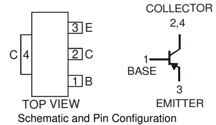
SOT89-3L
