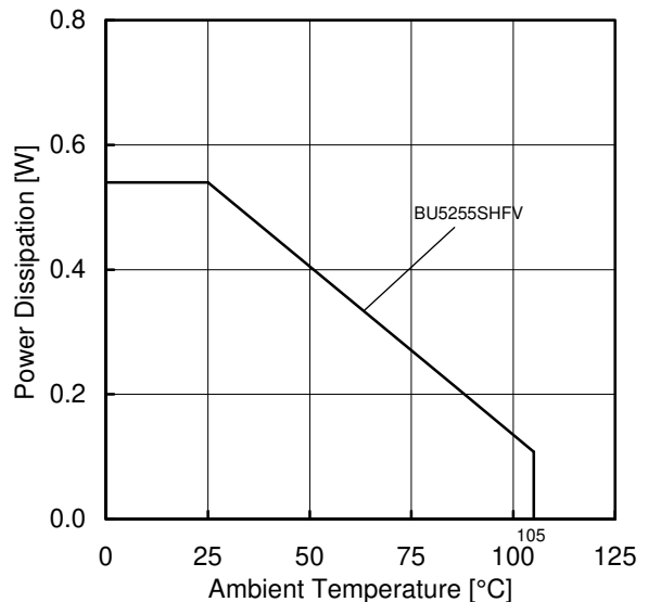
(d) BU5255SHFV
