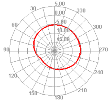
960.000MHz H
