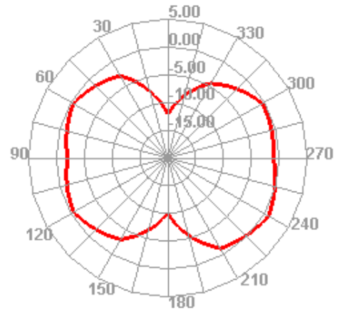
2700.000MHz E2
