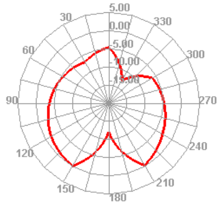
600.000MHz E2
