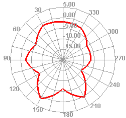
840.000MHz E2
