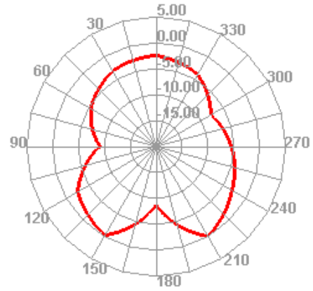
960.000MHz E2
