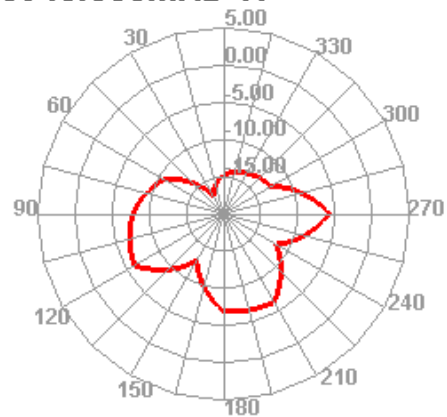
5940.000MHz H
