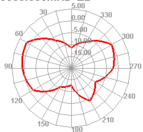
3300.000MHz E2
