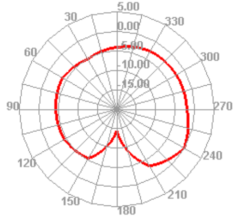
4980.000MHz H
