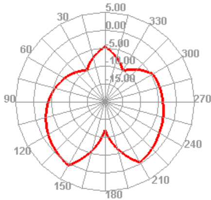
600.000MHz E1
