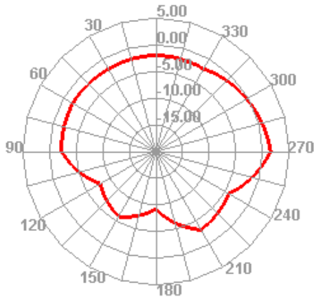
1560.000MHz E1
