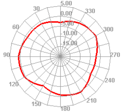
3300.000MHz H
