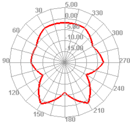
840.000MHz E1
