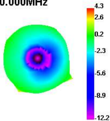
2700.000MHz
