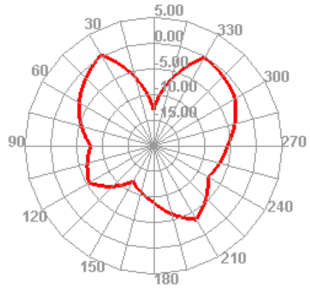
5940.000MHz E2
