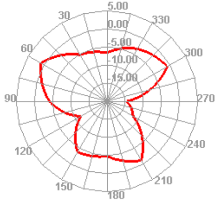
4980.000MHz E1
