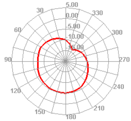
1200.000MHz H
