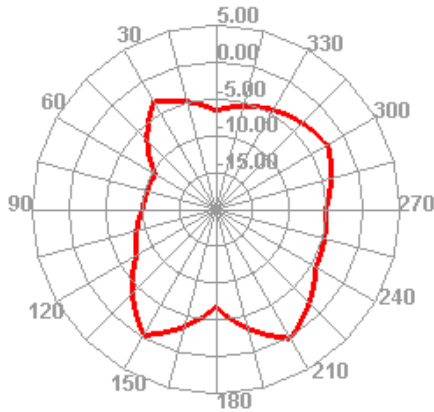
1200.000MHz E1
