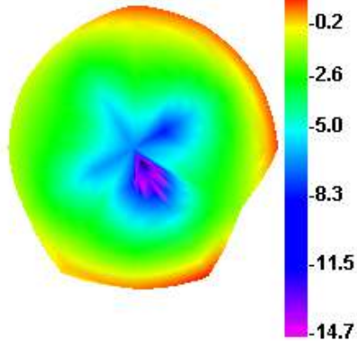
4980.000MHz
