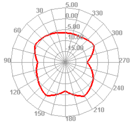
1200.000MHz E2
