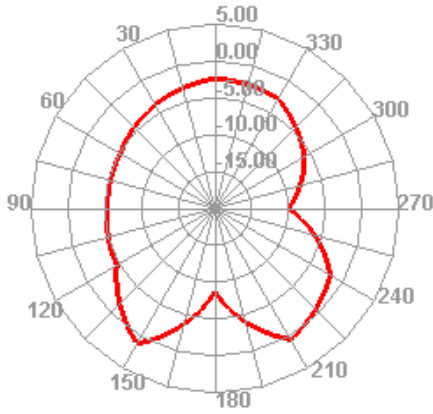
960.000MHz E1
