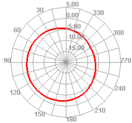
840.000MHz H
