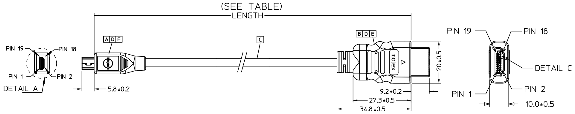
P1 HDMI D TYPE(M)
