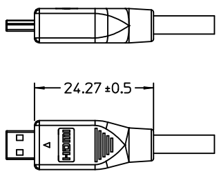
P1 HDMI D TYPE(M)
