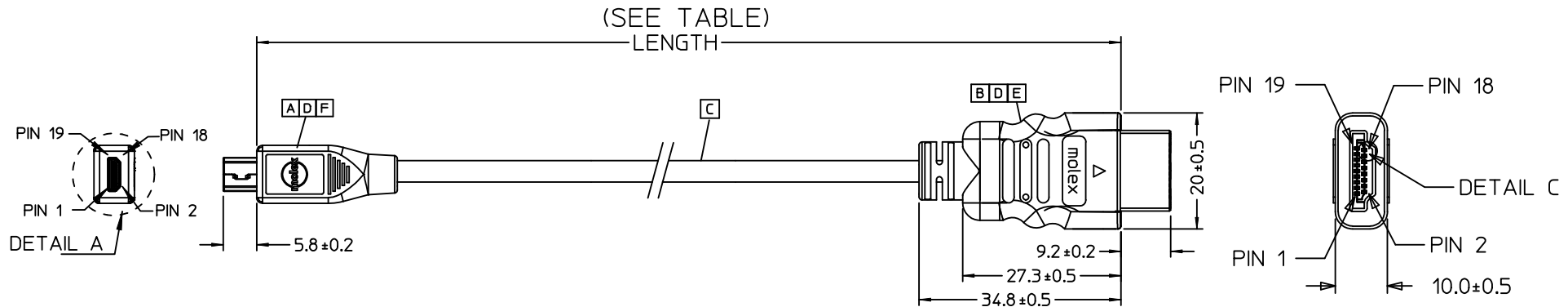
P1 HDMI D TYPE(M)
