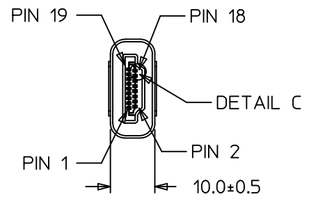
HDMI A TYPE(M) P2
