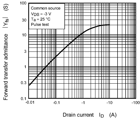
Fig. 7.7 |Y_{fs}| - I_D
