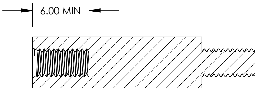
SECTION A-A SCALE 4 : 1
