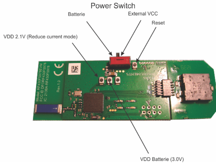
Figure 16. RF430F5978EVM Module
