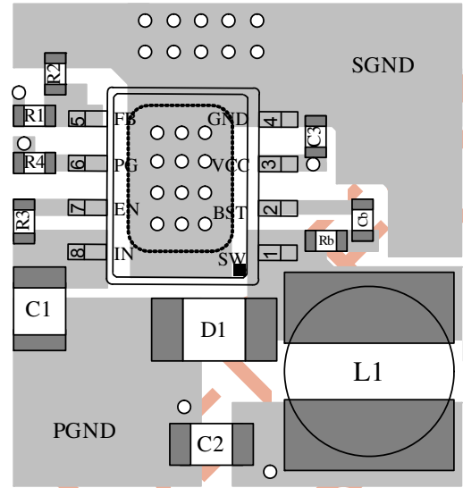
Top Layer
