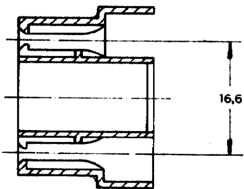
SEÇÃO A-A
