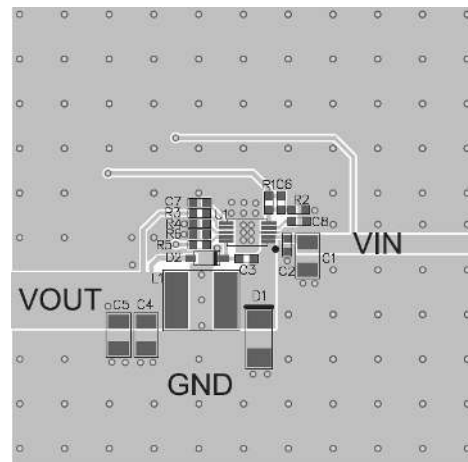
Top Layer
