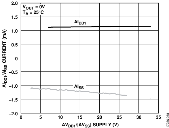
Figure 58. I_{DD1}/I_{SS} Current vs. AV_{DD1}/AV_{SS} Supply
