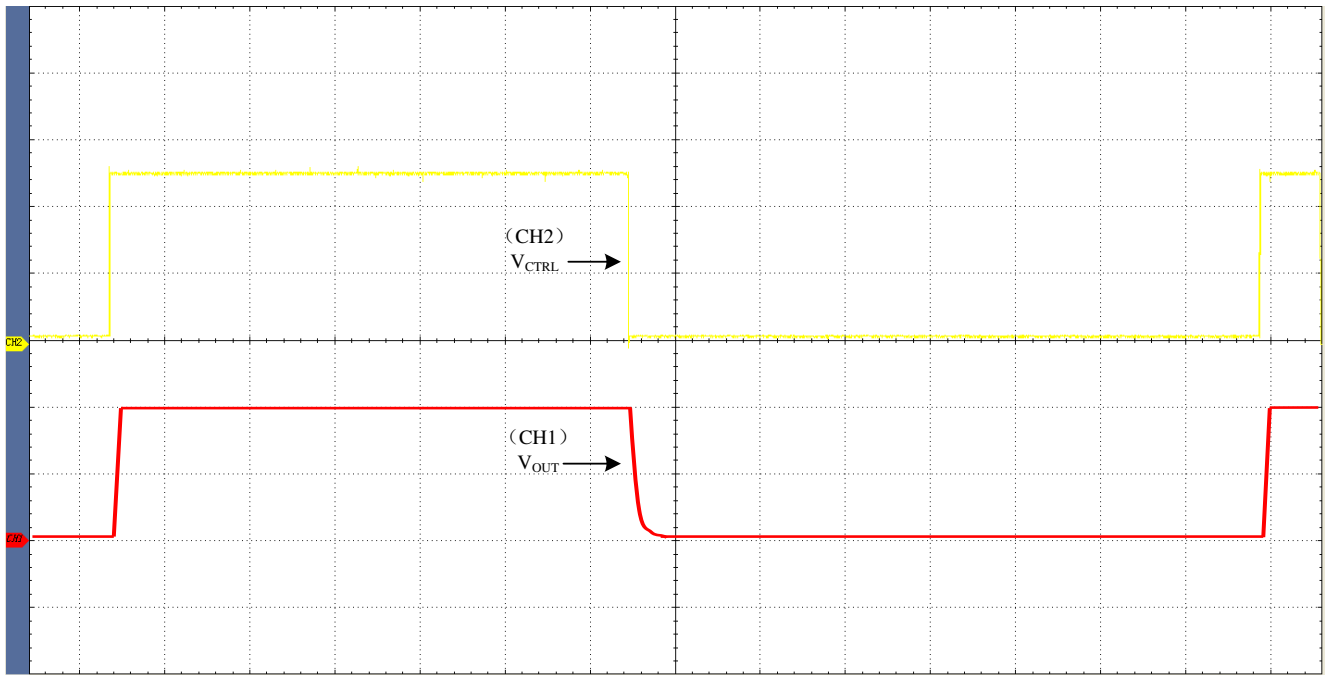
CH1: 10000V/Div CH2: 2V/Div M: 500ms V_{CTRL} : 0.25V ~ 5V V_{OUT} : 1000V ~ 20000V
