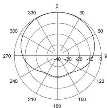
H-Plane | 405 MHz
