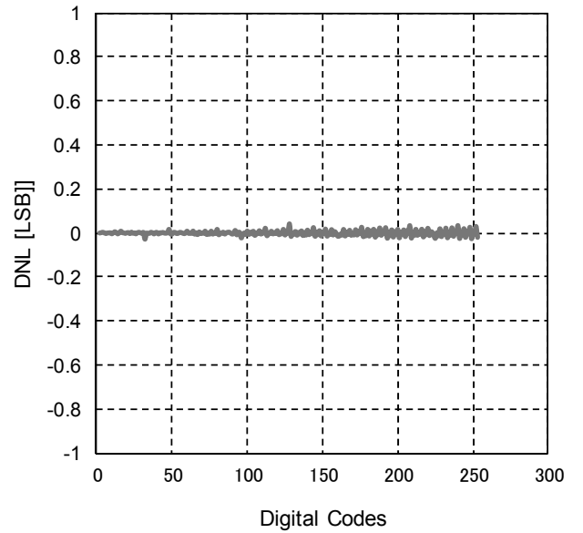
Fig.40 HAVDD DNL
