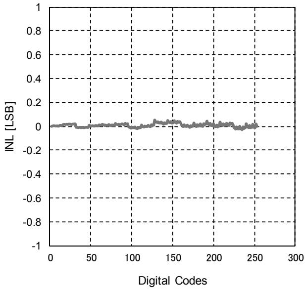
Fig.39 HAVDD INL
