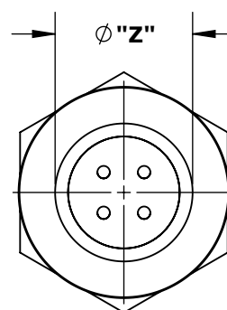
WIRING END W7381-4PG-P-3ES SHOWN
