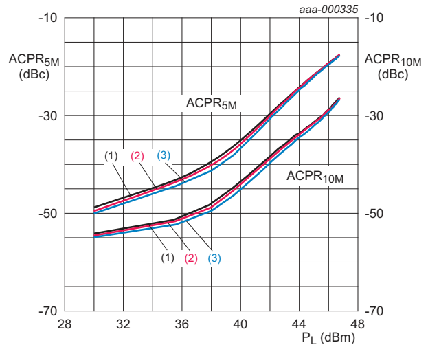
V_{DS} = 28\text{ V}; I_{Dq} = 410\text{ mA}. (1) f = 2115\text{ MHz} (2) f = 2140\text{ MHz} (3) f = 2165\text{ MHz}
