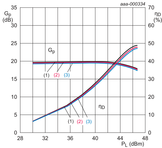
V_{DS} = 28\text{ V}; I_{Dq} = 410\text{ mA}. (1) f = 2115\text{ MHz} (2) f = 2140\text{ MHz} (3) f = 2165\text{ MHz}
