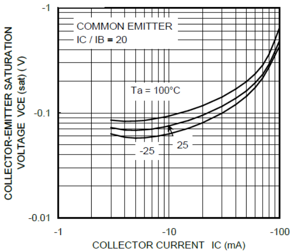
Fig. 10.18 RN2116 V_{CE(sat)} - I_C
