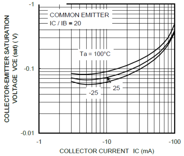
Fig. 10.17 RN2115 V_{CE(sat)} - I_C
