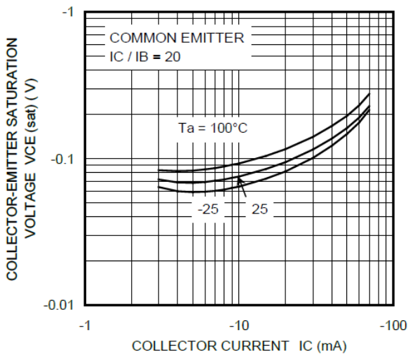
Fig. 10.18 RN2116 V_{CE(sat)} - I_C
