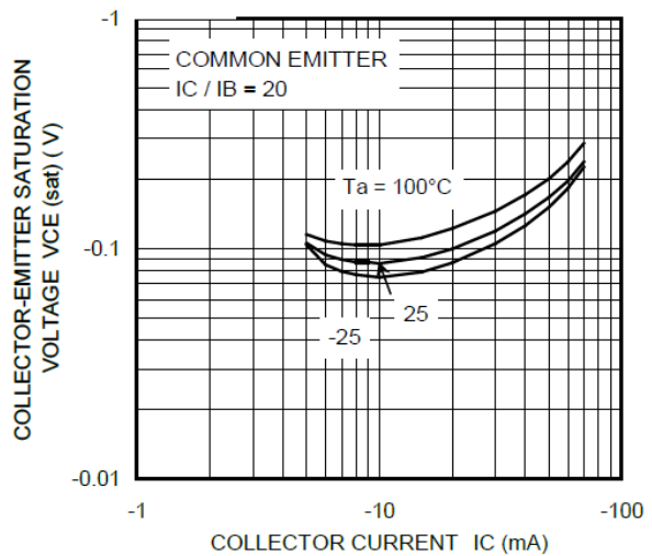
Fig. 10.19 RN2117 V_{CE(sat)} - I_C
