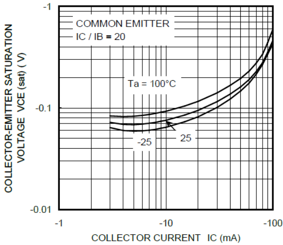
Fig. 10.16 RN2114 V_{CE(sat)} - I_C
