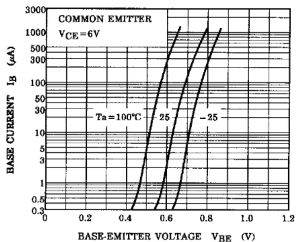
Fig. 8.6 I_B - V_{BE}
