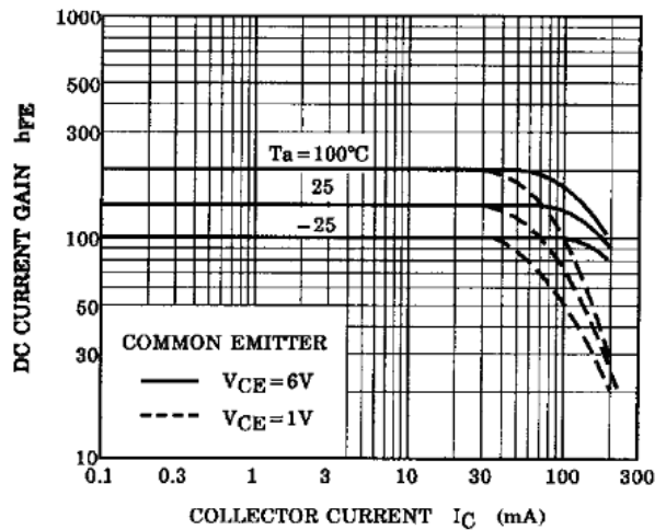
Fig. 8.2 h_{FE} - I_C
