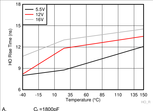
Figure 6-24. HO Rise Time
