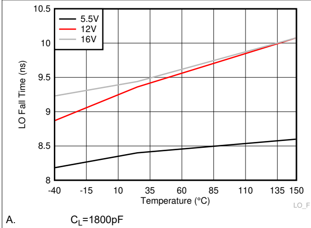
Figure 6-23. LO Fall Time
