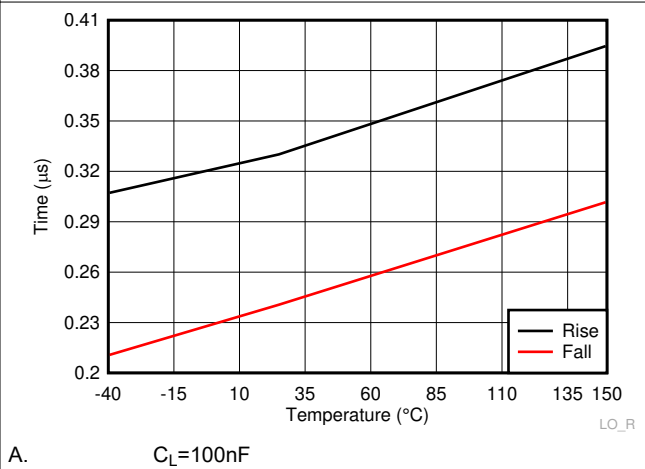
Figure 6-26. LO Rise & Fall Time
