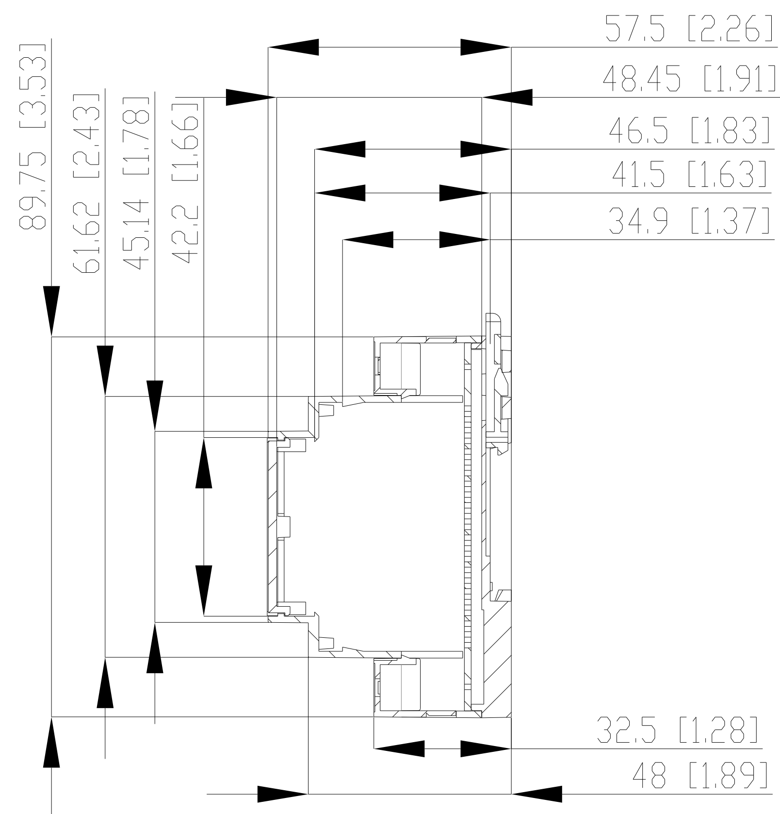
SECTION B-B SCALE 2 : 3
