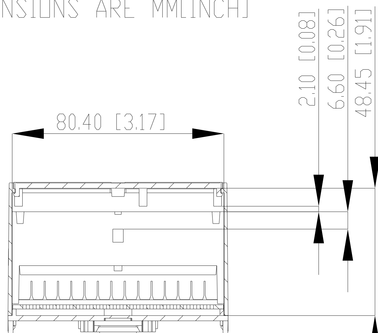
SECTION D SCALE 2 : 1
