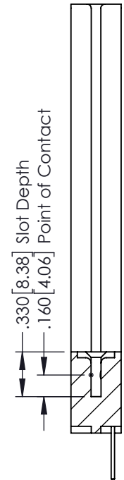
SECTION A-A
