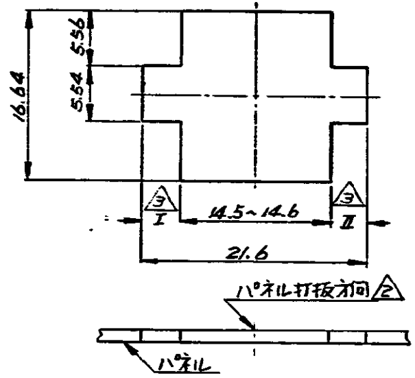
取付穴寸法(寸法公差±0.1) 尺度 2-1
