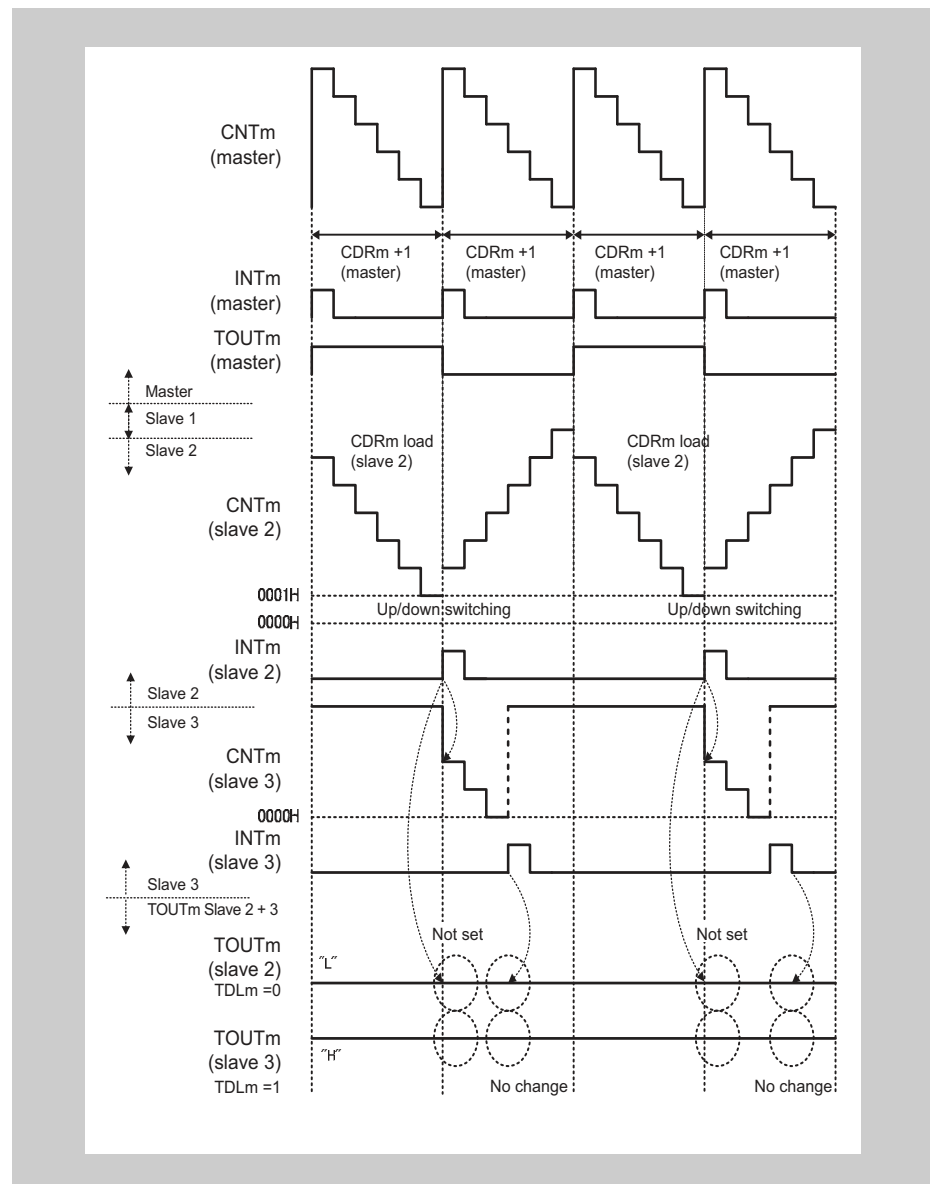
Figure 14-92 TAUBnCDRm \text{ (slave)} \geq TAUBnCDRm \text{ (master)} + 1
