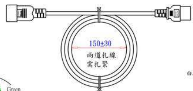
A-CI 扎線圖示 (A-CI Hank Detail)
