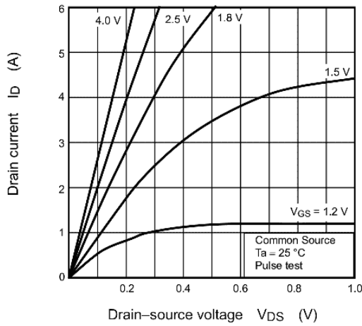
Fig. 7.1 I_D - V_{DS}
