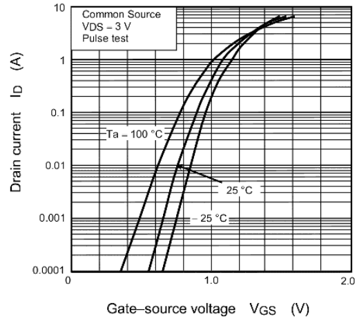
Fig. 7.2 I_D - V_{GS}
