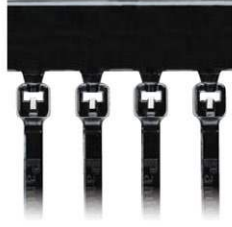
BT_XMR (0, 30)
