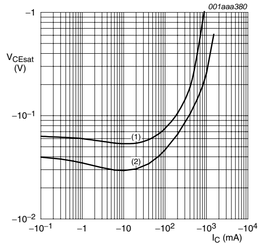
T_{amb} = 25\text{ }^\circ\text{C} (1) I_C/I_B = 50 (2) I_C/I_B = 20
