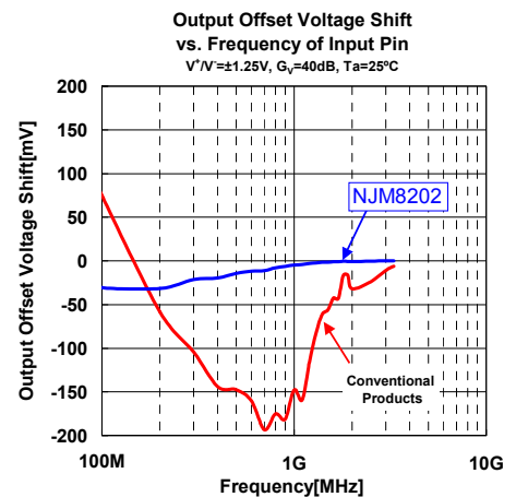
NJM8202RB1 (MSOP8(TVSP8))
