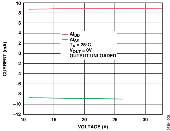
Figure 67. I_{DD}/I_{SS} vs. A_{VDD}/A_{VSS}
