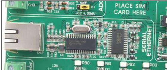
Figure 8-1: Ethernet module
