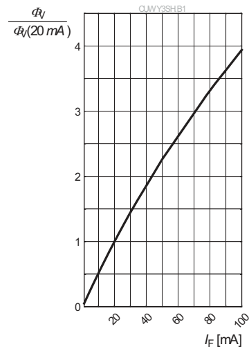
Relative Luminous Flux 6) page 22 Relativer Lichtstrom 6) Seite 22 \Phi_V / \Phi_V(20\text{ mA}) = f(I_F); T_S = 25\text{ °C}
