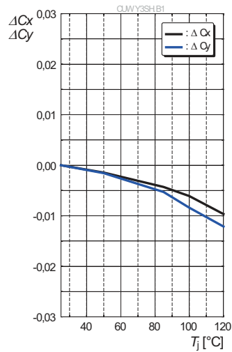
Chromaticity Coordinate Shift 6) page 22 Farbortverschiebung 6) Seite 22 \Delta C_x, \Delta C_y = f(T_j); I_F = 20 \text{ mA}
