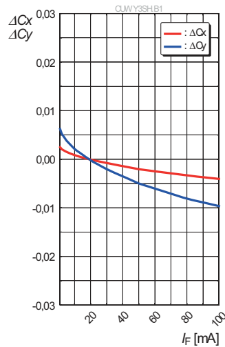
Chromaticity Coordinate Shift 6) page 22 Farbortverschiebung 6) Seite 22 \Delta C_x, \Delta C_y = f(I_F); T_S = 25\text{ °C}
