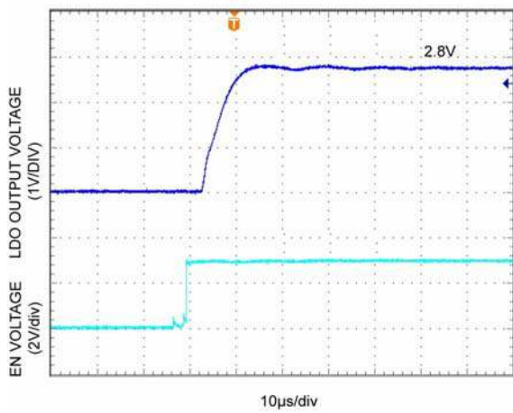
LDO Enable
