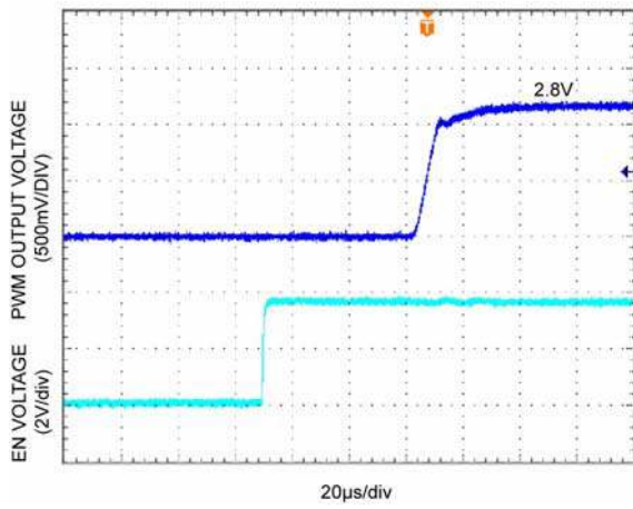
DC-DC Enable
