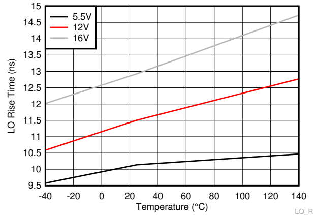
Figure 6-22. LO Rise Time
