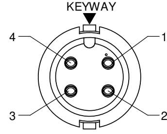
FACE VIEW P/N: 6282-4SG-3XX
