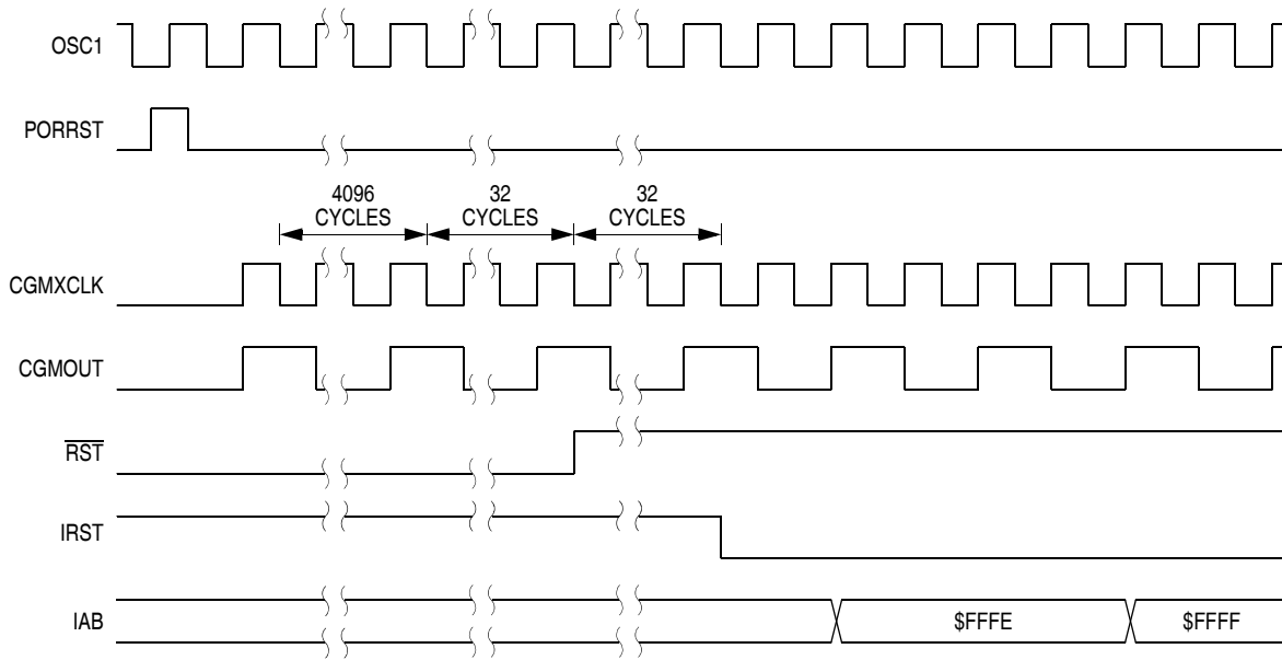
Figure 14-7. POR Recovery
