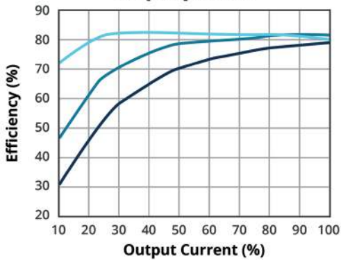
EFFICIENCY VS OUTPUT LOAD PDQ10-Q24-S3-D
