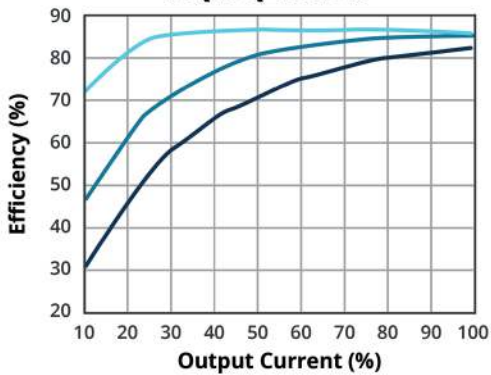
EFFICIENCY VS OUTPUT LOAD PDQ10-Q24-S15-D
