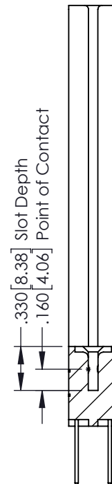
SECTION A-A
