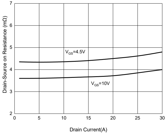
Fig. 3 - R_{DS(ON)} - I_D
