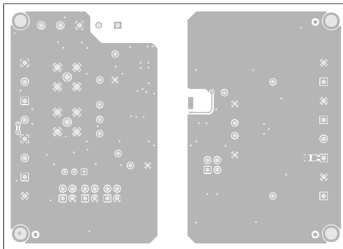
Figure 8. EVAL-ADM3055EBZ Bottom Layer
