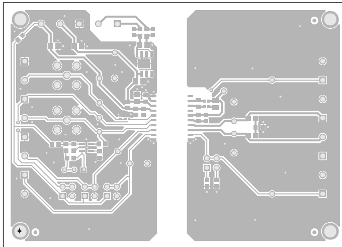
Figure 7. EVAL-ADM3055EBZ Top Layer
