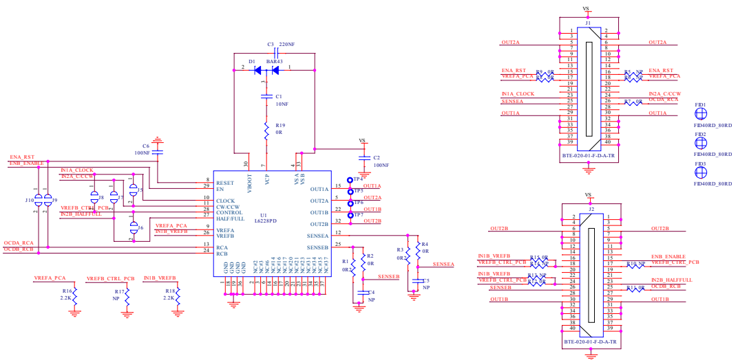
Figure 9. EVL6228-PLUG
