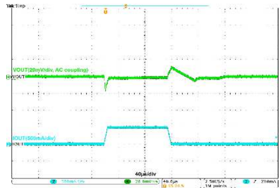
Figure 19. LDO1/2 Load Transient, V_{\text{IN}} = 1.3\text{ V} , V_{\text{OUT}} = 1.05\text{ V} , 1\text{ mA} \leftrightarrow 500\text{ mA} , 5\text{ }\mu\text{s} Edge
