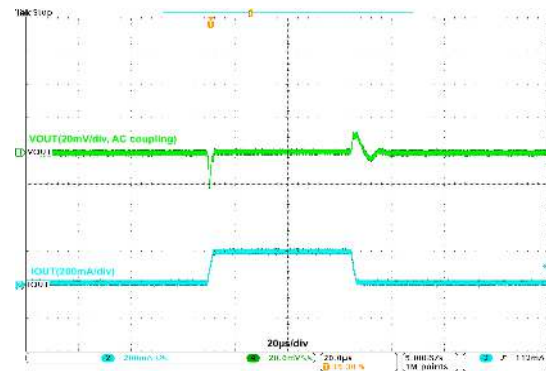
Figure 21. LDO5 Load Transient, V_{\text{IN}} = 2.05\text{ V} , V_{\text{OUT}} = 1.8\text{ V} , 1\text{ mA} \leftrightarrow 200\text{ mA} , 2\text{ }\mu\text{s} Edge
