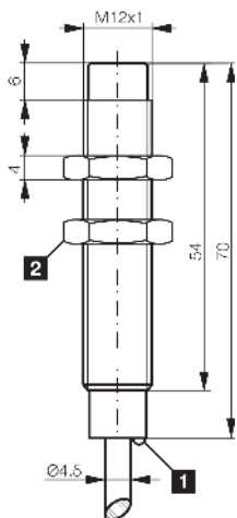
1) LED 2) Schlüsselweite 17 mm
