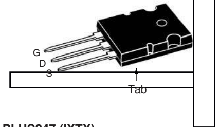
PLUS247 (IXTX)
