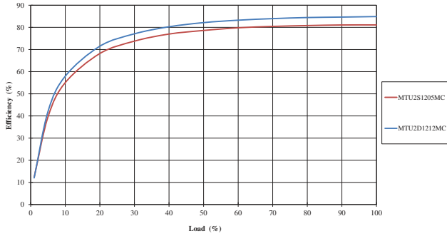
12V INPUT
