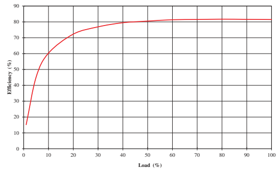
24V INPUT
