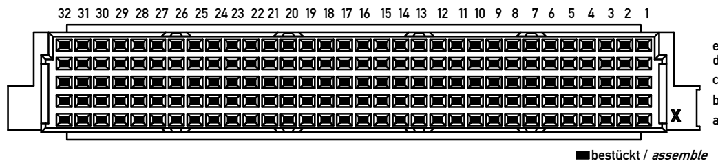
Leiterplatten-Lochbild / PCB drillhole pattern
