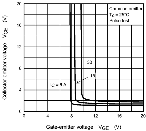
Fig. 8.3 V_{CE} - V_{GE}
